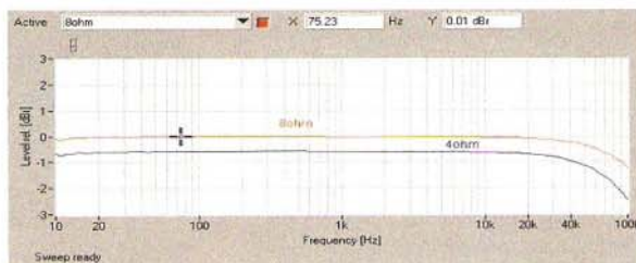
Rys. 1. Pasma przenoszenia
