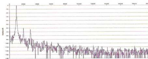
Rys. 2. Zniekształcenia harmoniczne
